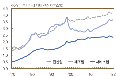
〈그림 21〉 자본집약도(K/Y)
