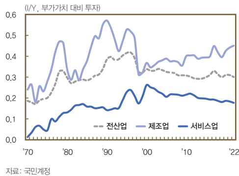
〈그림 22〉 투자율(I/Y)
